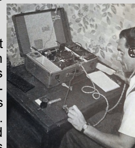
Un opérateur radio avec son poste qui tient dans une valise
